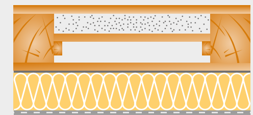
Unterdeckendämmung
