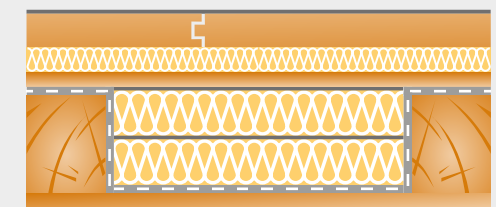
Zwischendeckendämmung
