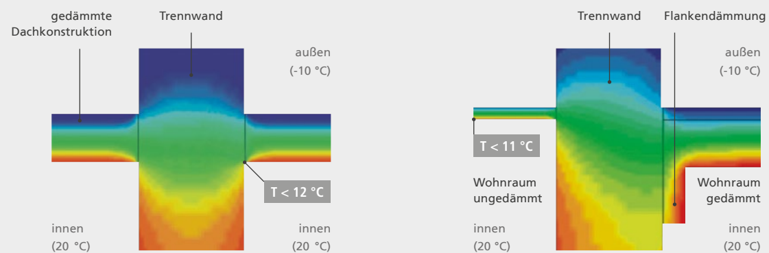
Ungedämmte Haustrennwand
