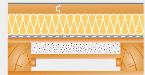
Aufdeckendämmung
