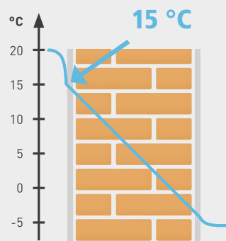
365 mm Ziegelwand ohne Dämmung
